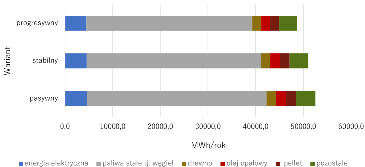
Rysunek 39. Perspektywiczne zużycie energii z podziałem na poszczególne rodzaje paliw i nośników energii dla roku 2036 źródło: opracowanie własne
