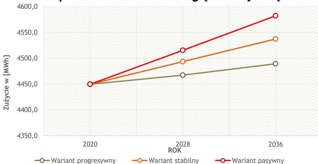
Rysunek 35. Prognozowana zmiana rocznego zużycia energii elektrycznej do roku 2036
